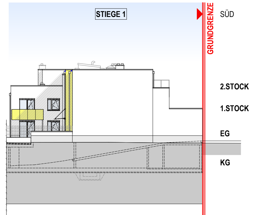
STIEGE 1, ANSICHT WEST M = 1:300
