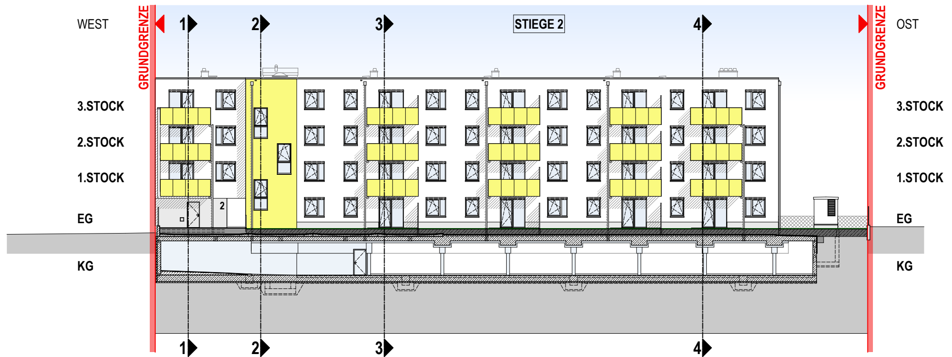
STIEGE 2, ANSICHT SÜD M = 1:300
