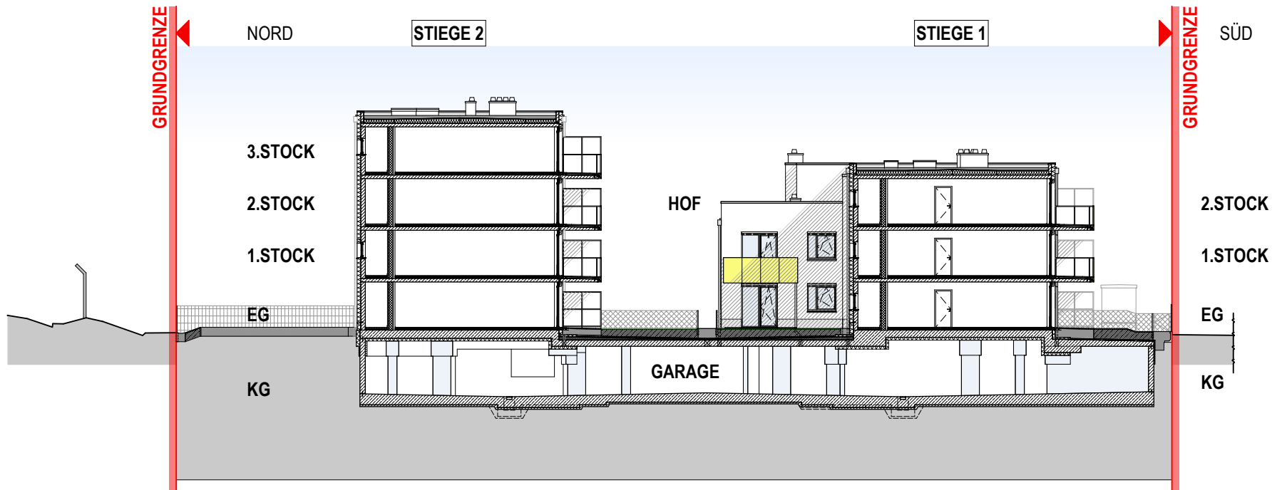
SCHNITT 3-3 M = 1:300
