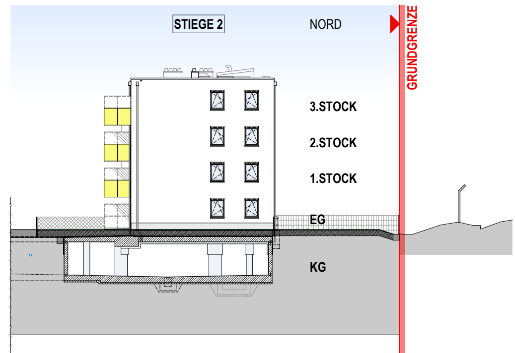
STIEGE 2, ANSICHT OST M = 1:300
